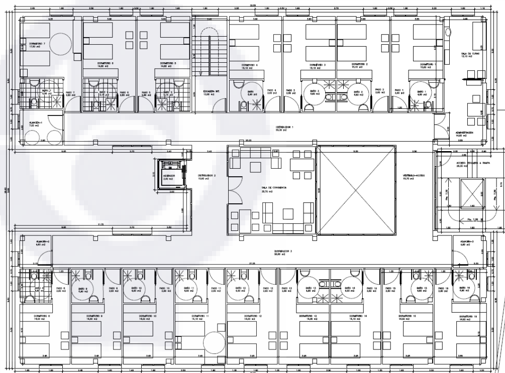
PLANTA ALTA - RESIDENCIA
