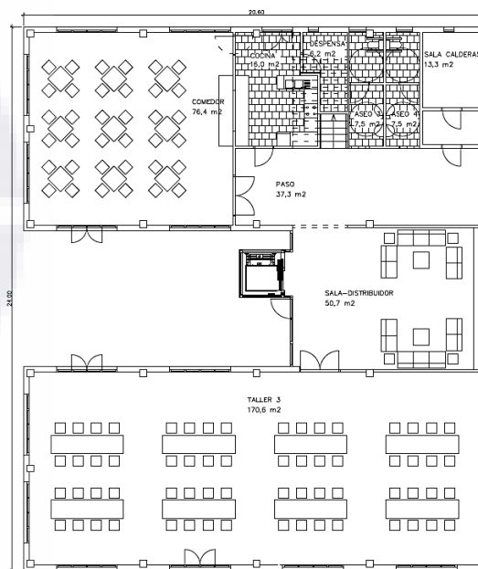
PLANTA SEMISÓTANO
